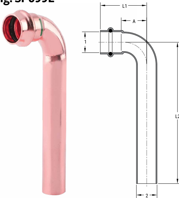
SP699L CU P X MS EXTND STREET 90 ELL
