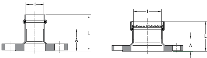
SP616 CU FLNG ADPTR, 4-BOLT
