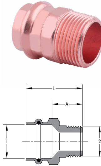
SP607R P X MT RED ADPT CPLG
