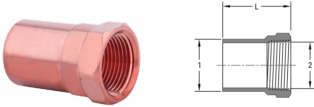
SP603 MS x FT ADPT CPLG
