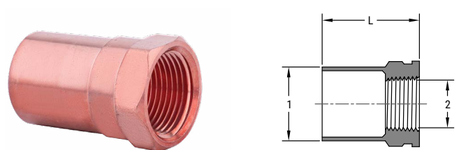
SP603R MS x FT ADPT CPLG
