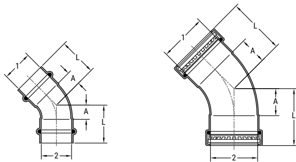
SP645 CU P X P 45 ELL
