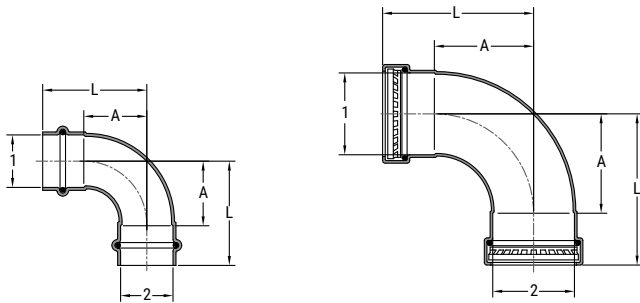
SP690 CU P X P 90 ELL
