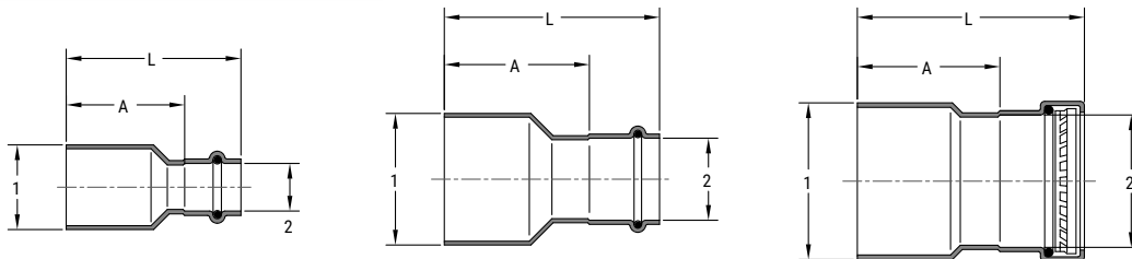
SP609R CU MS X P RED ADPT CPLG
