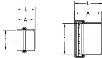
SP600 CU END CAP
