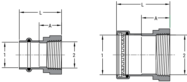
SP608 CU P X FT ADPT CPLG
