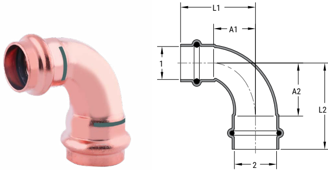
SP690R CU P X P RED 90 ELL
