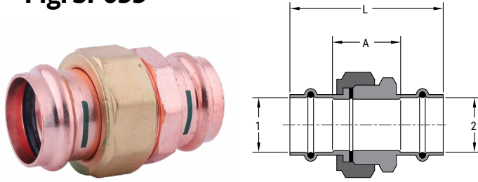
SP655 CU P X P EPDM UNION
