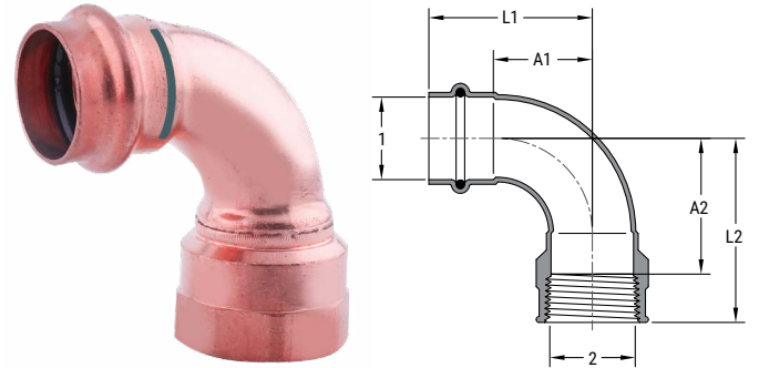
SP698 CU P X FT 90 ELL
