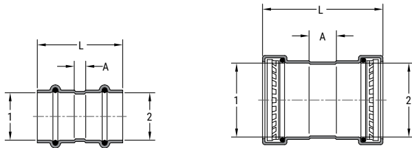
SP604 CU P X P COUPLING
