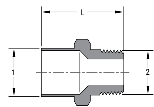
SP602R MS X MT RED ADPT CPLG
