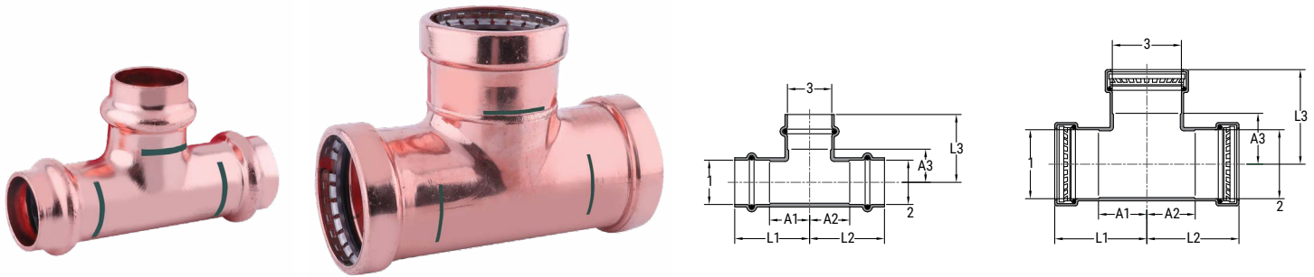
SP690 CU P x P x P Tee
