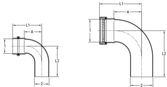
SP699 CU P X MS STREET 90 ELL
